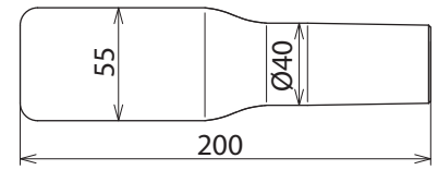
Maßbild FD 55 NS
