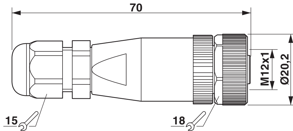
Maßzeichnung
