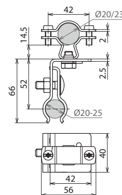
Maßbild DLH RSF ZS 20 23 V2A
