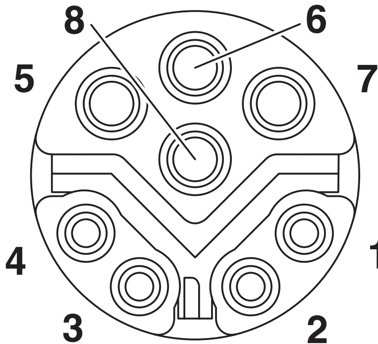
Plano esquemático
