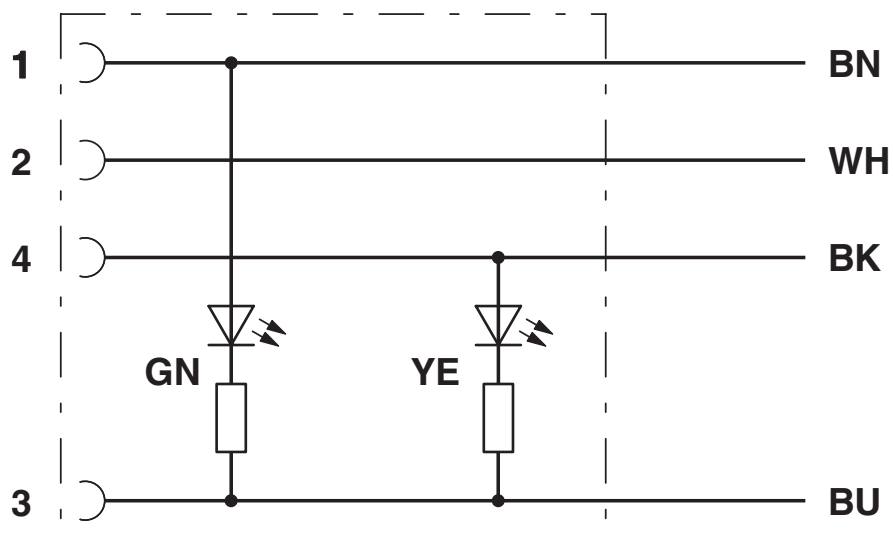
Kontaktbelegung der M8-Buchse mit LED
