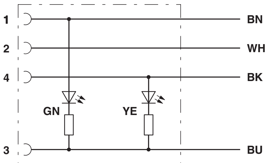
Diagrama eléctrico
