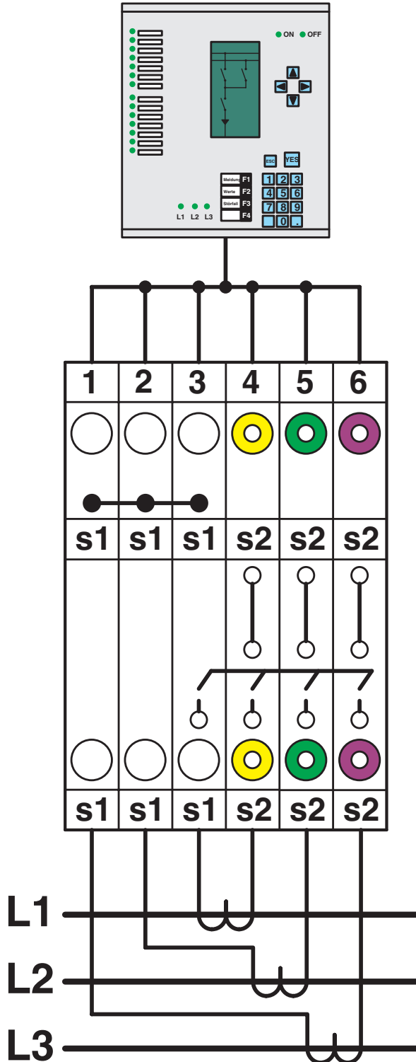
Plano esquemático
