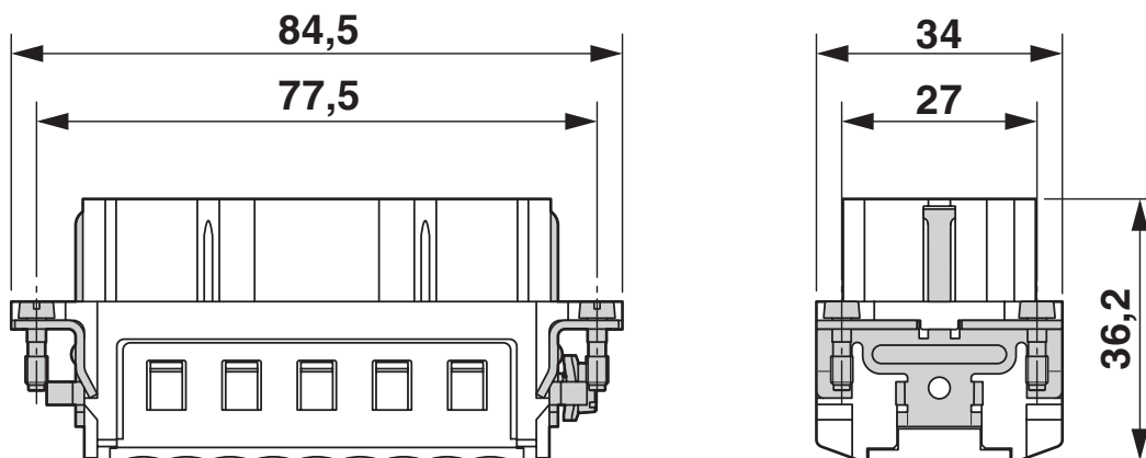
Dessin coté
