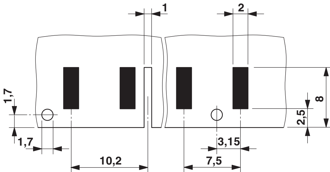
Gabarit perçage / géom. pastille soudage
