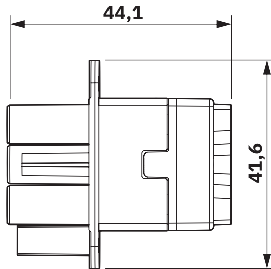
Maßzeichnung
