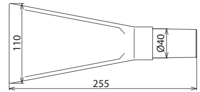
Maßbild FD 110 MS
