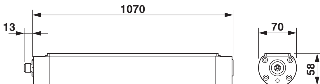
Esquema de dimensiones
