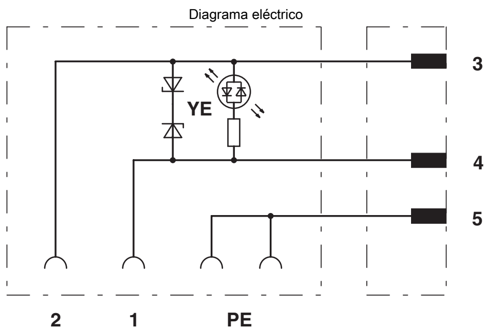
Ocupación de contactos del conector enchufable M12 y del conector de válvula
