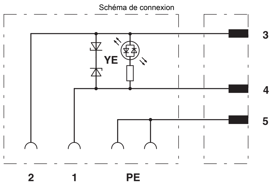
Affectation des contacts des connecteurs M12 mâles et du connecteur pour électrovanne
