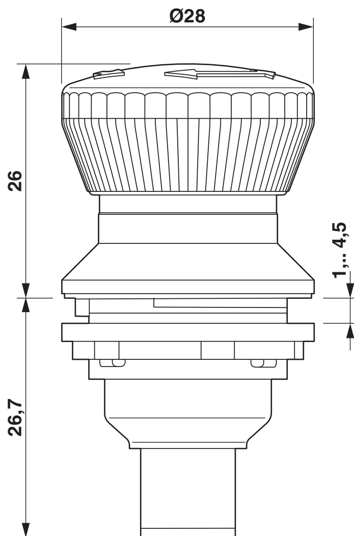
Dessin coté
