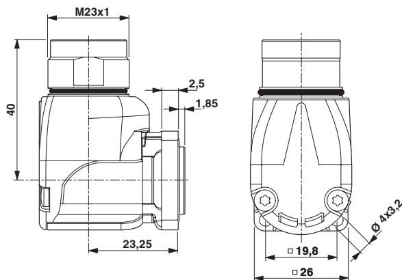
Dessin coté
