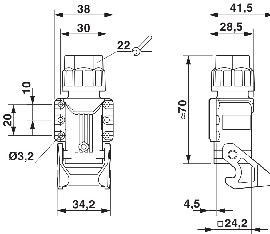
Maßzeichnung
