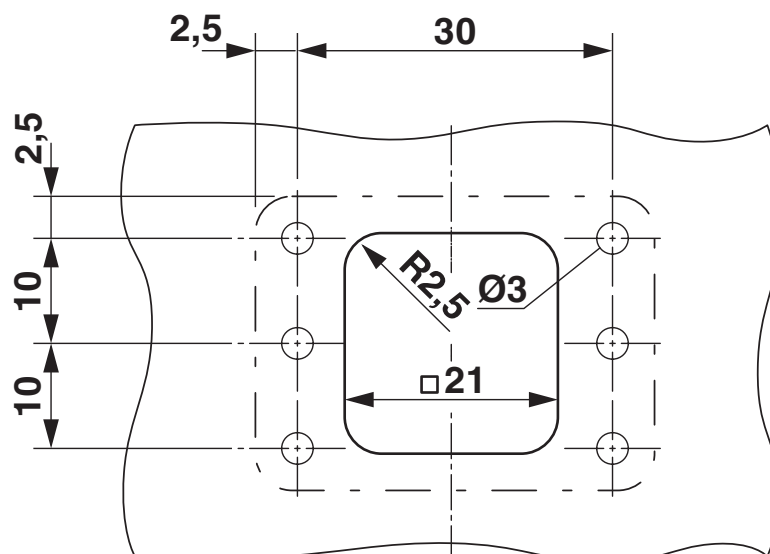
Maßzeichnung
