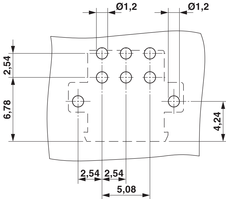
Esquema de taladros/geometría pads soldadura
