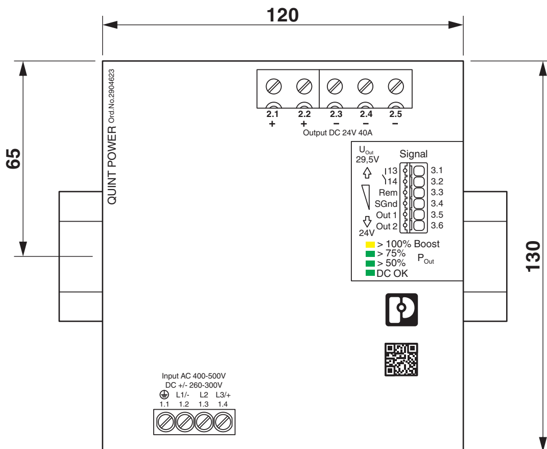
Maßzeichnung
