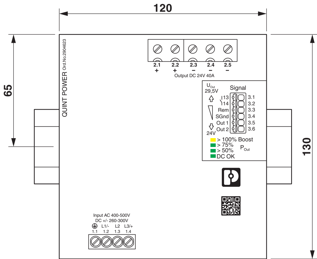
Dimensions vue de face (en mm)
