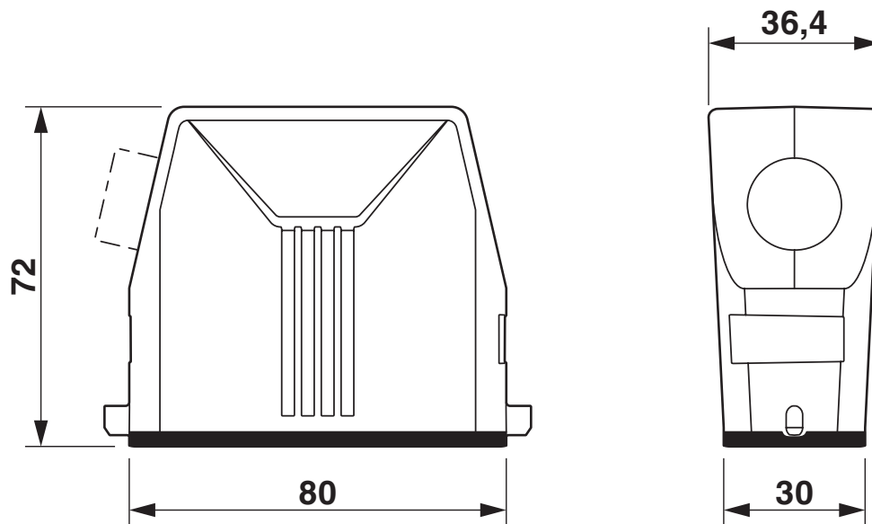
Maßzeichnung
