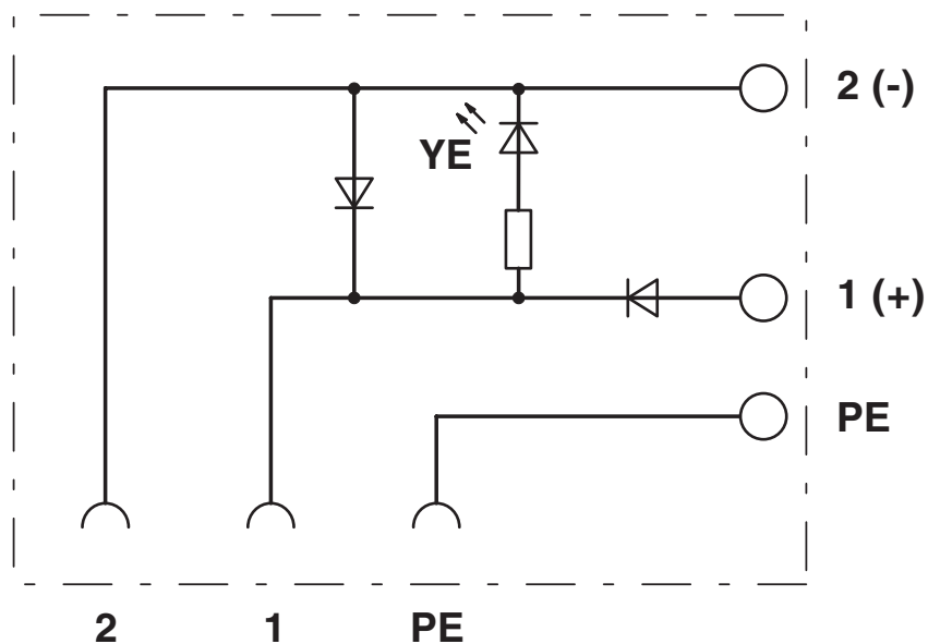
Diagrama eléctrico
