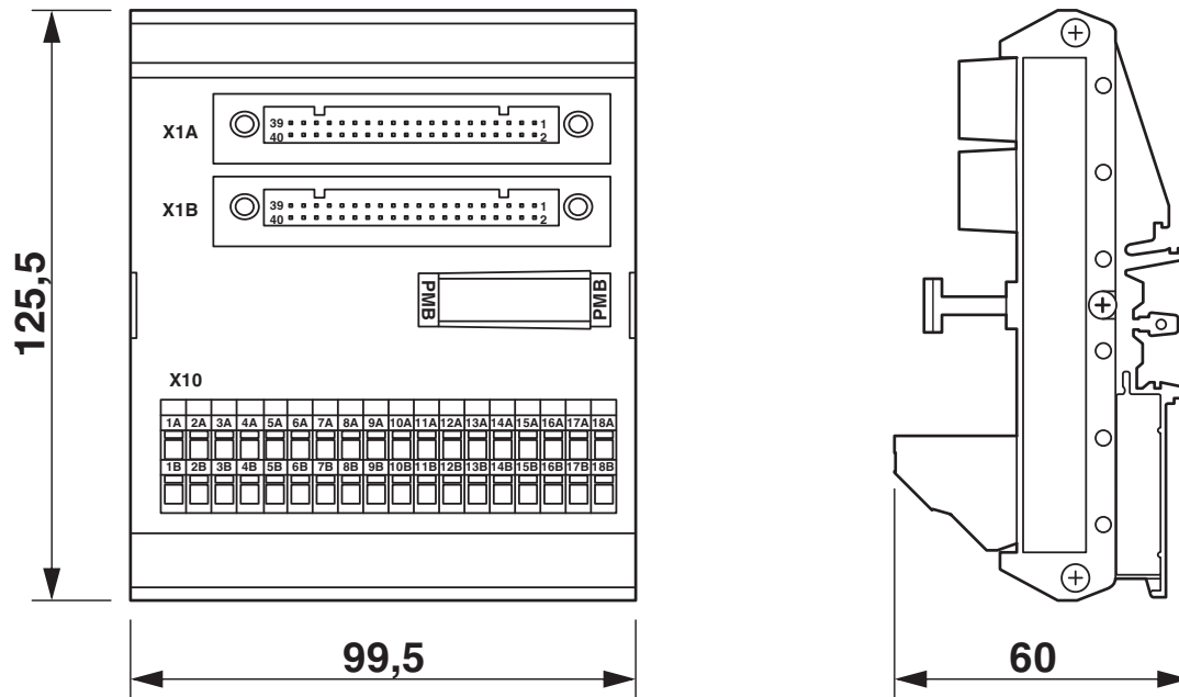
Maßzeichnung
