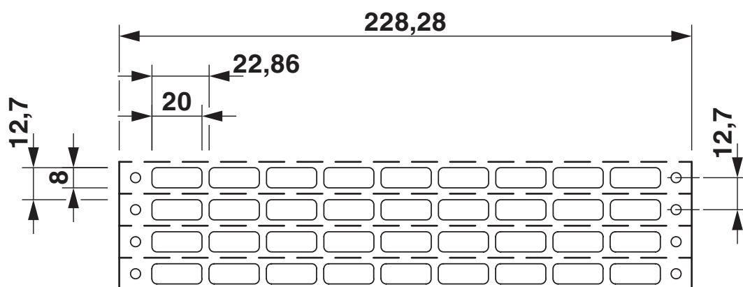
Dessin coté
