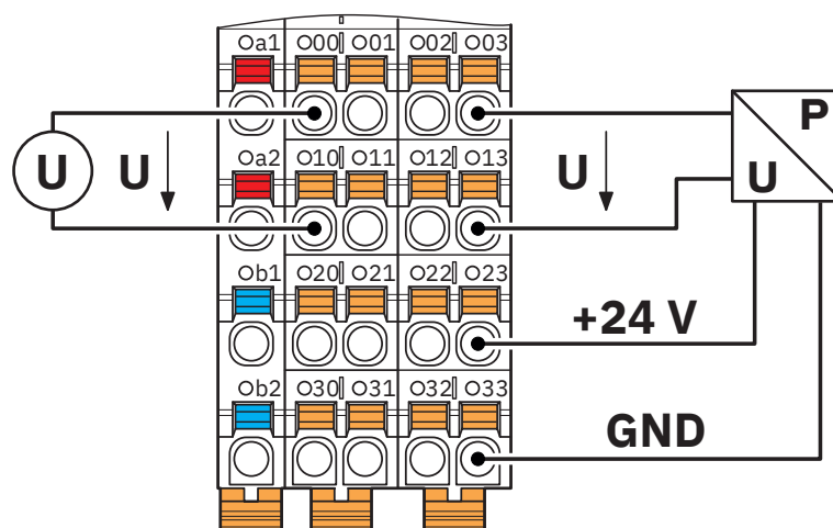
Dibujo de conexión
