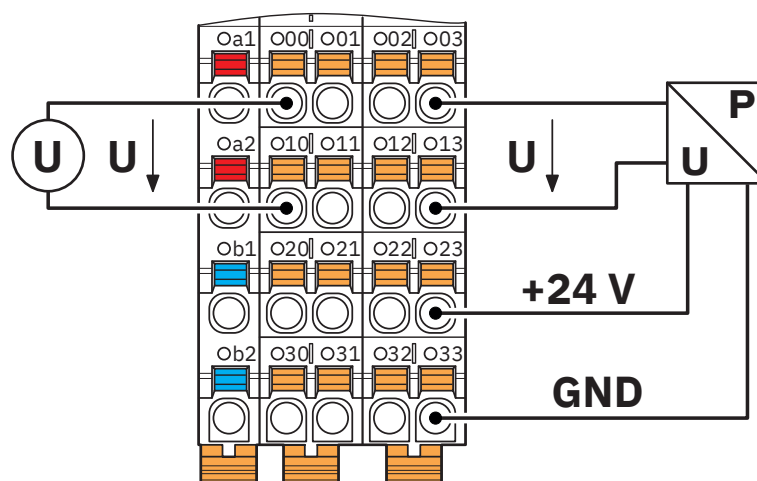
Dessin de la connexion
