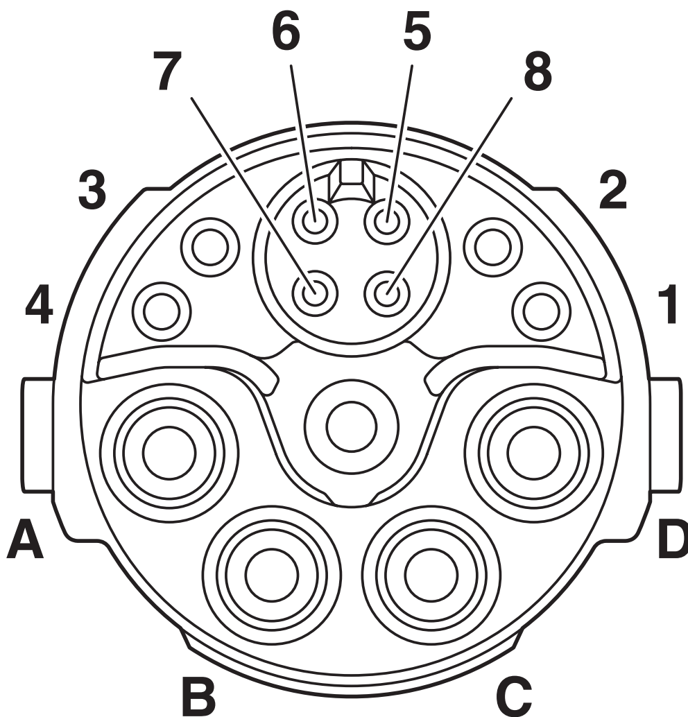
Esquema de polos conector hembra señal
