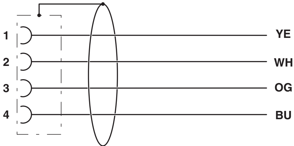
Kontaktbelegung der M12-Buchse
