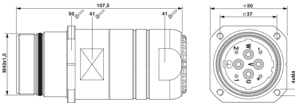
Dessin coté
