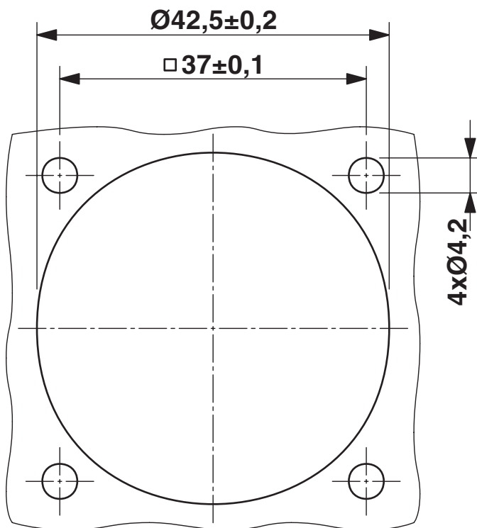
Dessin coté
