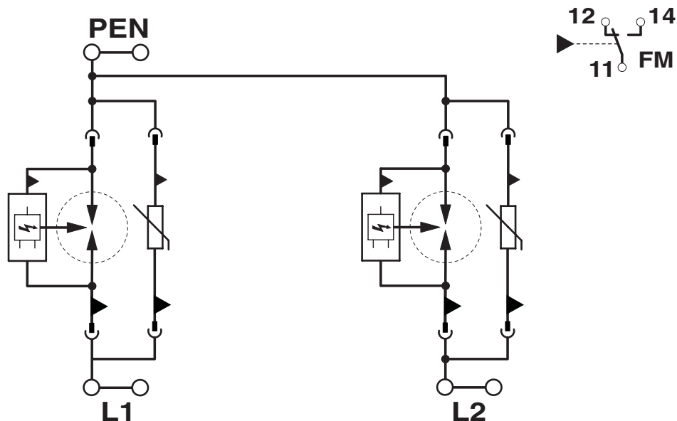
Diagrama eléctrico
