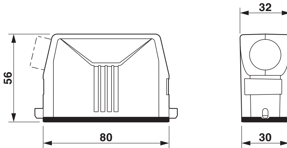
Maßzeichnung
