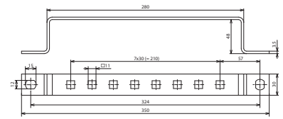
Maßbild ES 8AP 11X11 V2A
