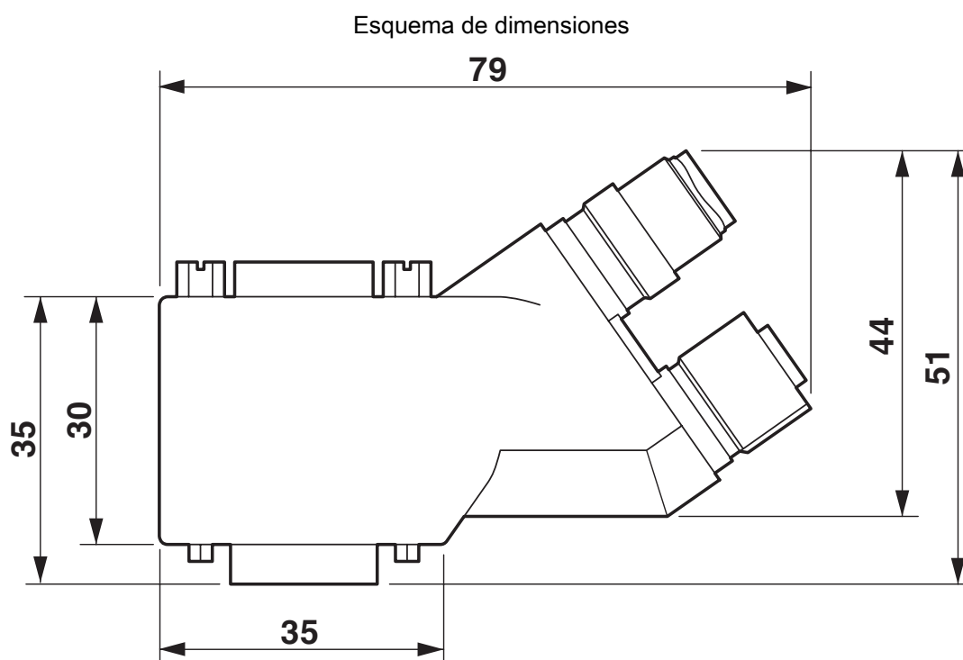
Esquema de dimensiones SUBCON-PLUS...35...M12, variante de 35°
