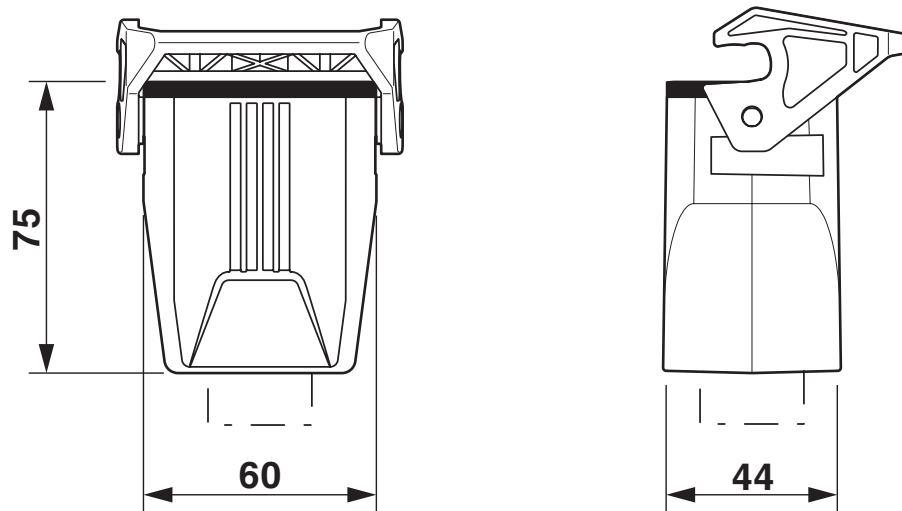
Maßzeichnung
