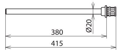
Maßbild L72 PS PHE 405
