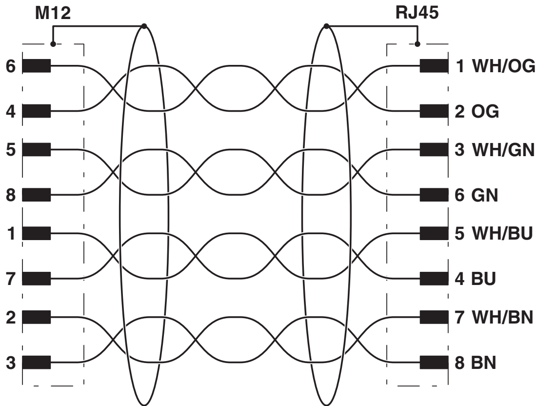
Schaltplan
