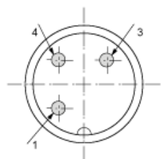
Connettore M12
