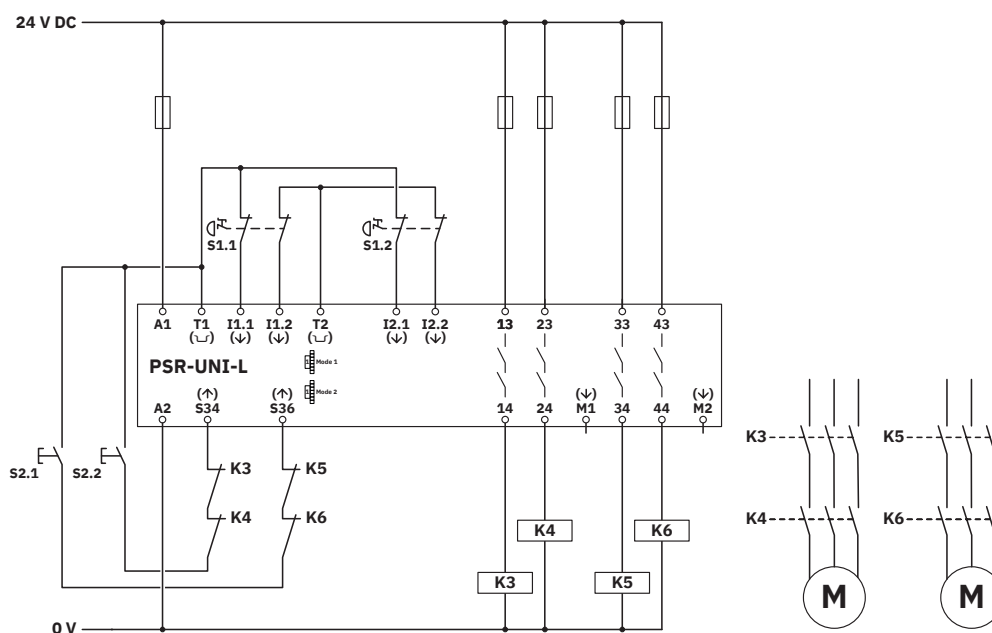
Diagrama eléctrico
