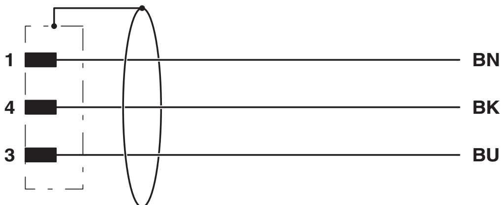
Ocupación de contactos del conector macho M8
