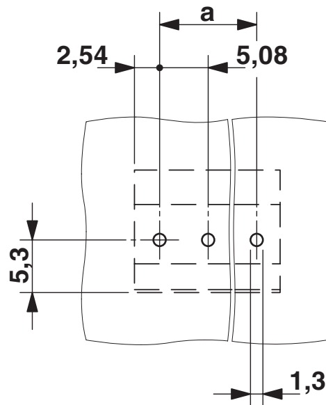
Bohrplan/Lötpadgeometrie
