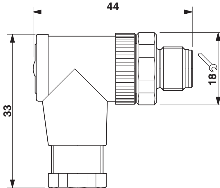
Maßzeichnung
