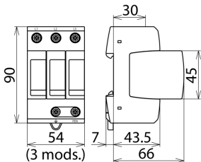
Dimensiones del DG M TNC 385
