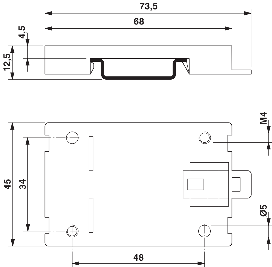
Maßzeichnung
