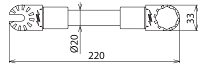
Maßbild ISV 220 ZK MS
