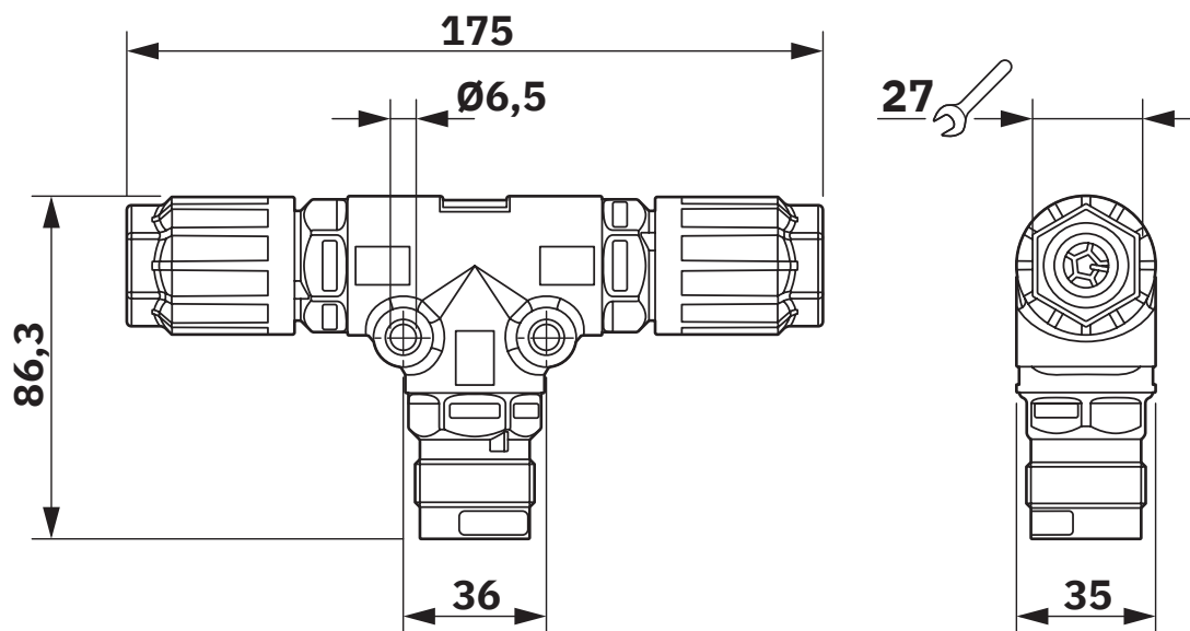
Dessin coté
