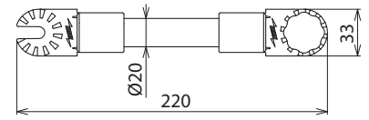
Maßbild ISV 220 ZK 123 SN7739
