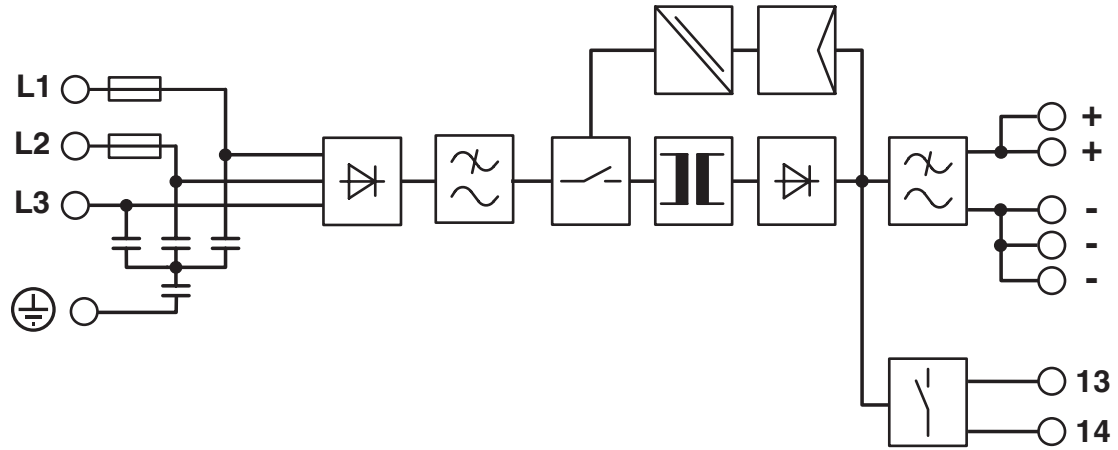
Schéma fonctionnel
