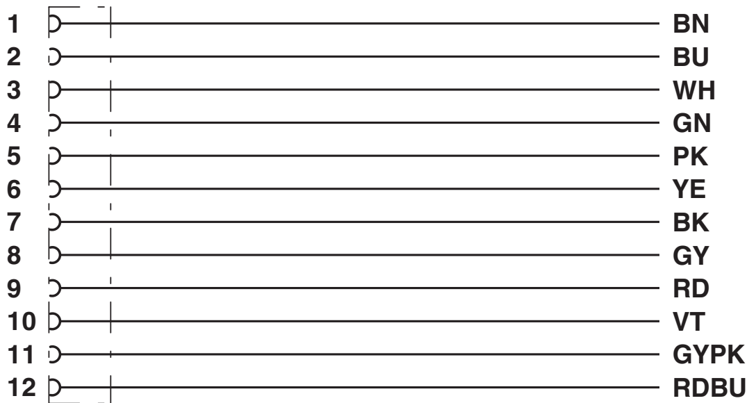
Diagrama eléctrico
