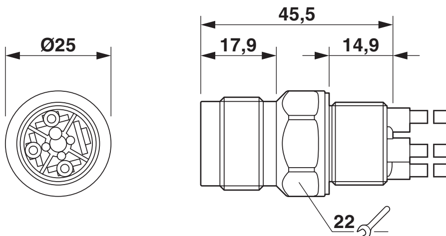
Maßzeichnung
