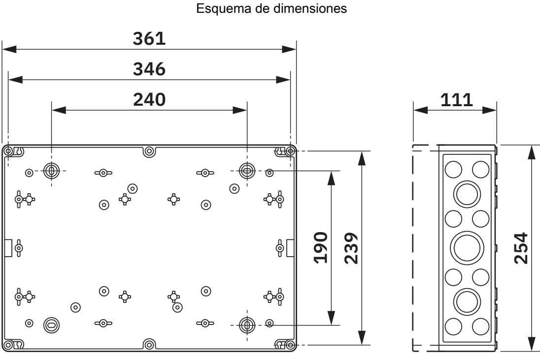
Dimensiones de la carcasa
